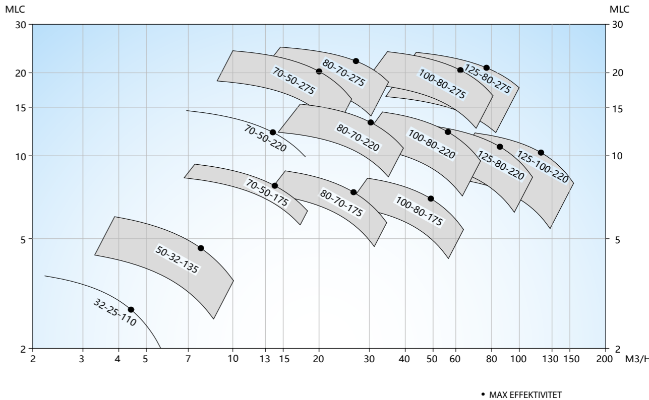
S Centrifugalpumpe, 1450 o/min., 50 Hz
