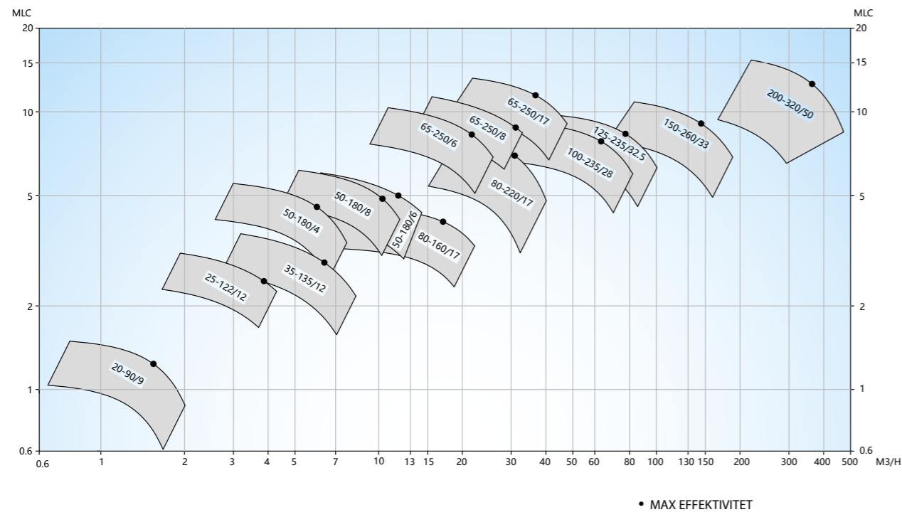
SA Centrifugalpumpe, 1152 o/min., 60 HZ
