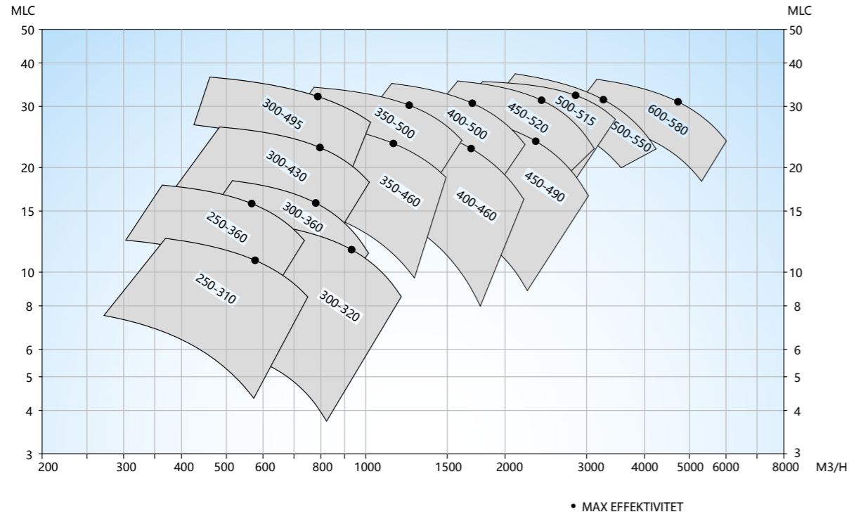
DSL Centrifugalpumpe, 960 o/min., 50 Hz
