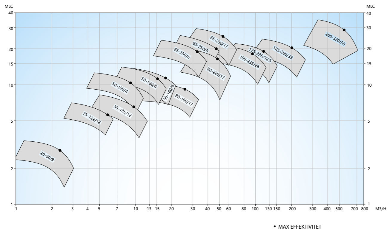
SA Centrifugalpumpe, 1740 o/min., 60 HZ
