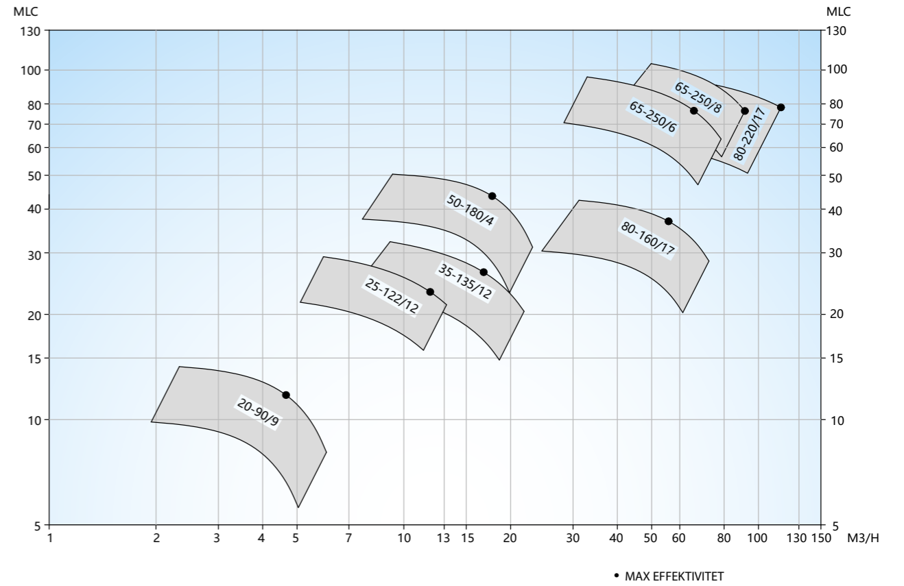
SA Centrifugalpumpe, 3450 o/min., 60 HZ
