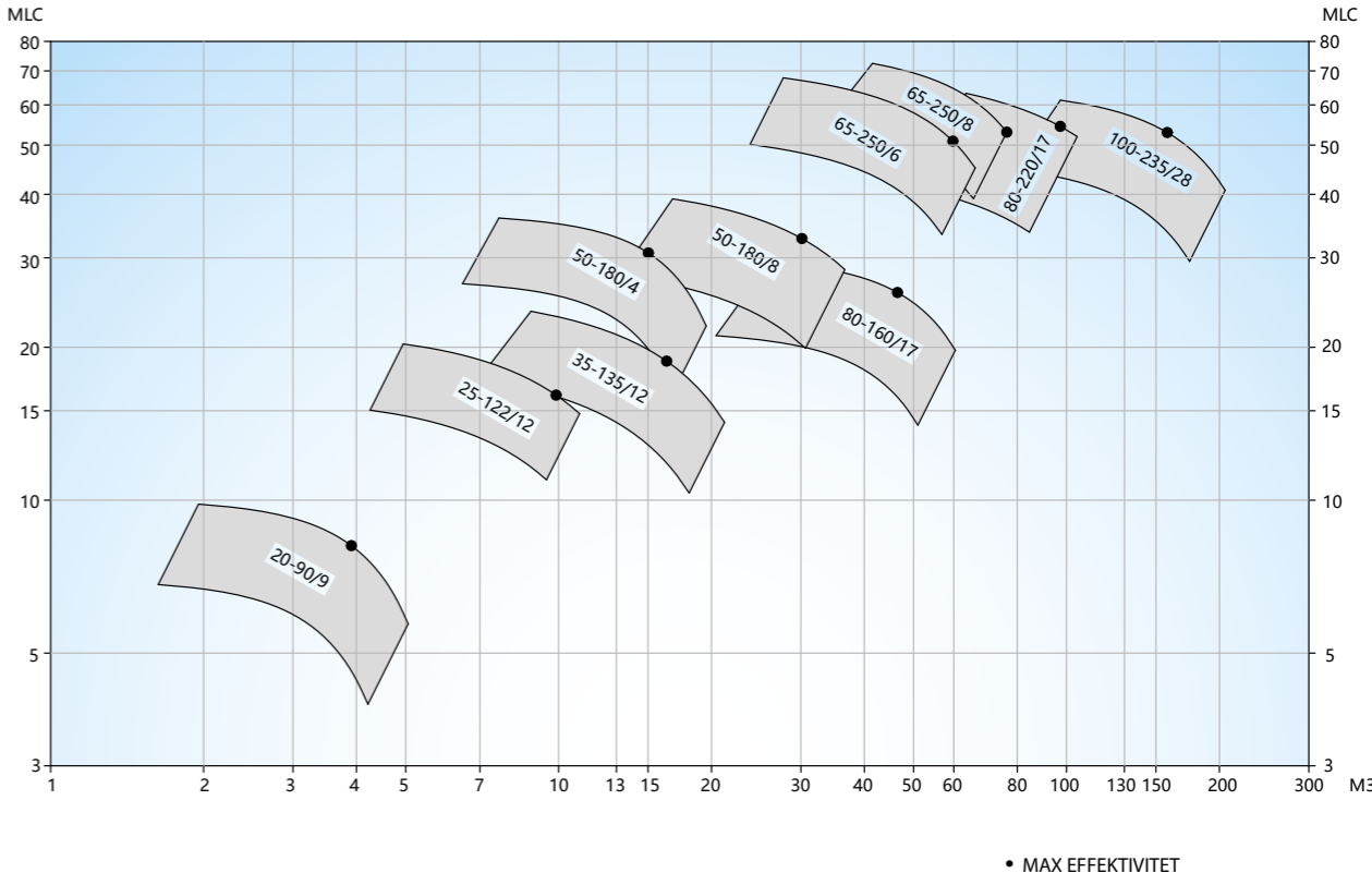
SA Centrifugalpumpe, 2950 o/min., 50 Hz
