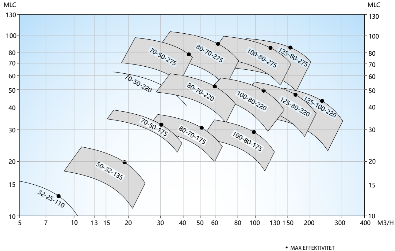
S Centrifugalpumpe, 2950 o/min., 50 Hz
