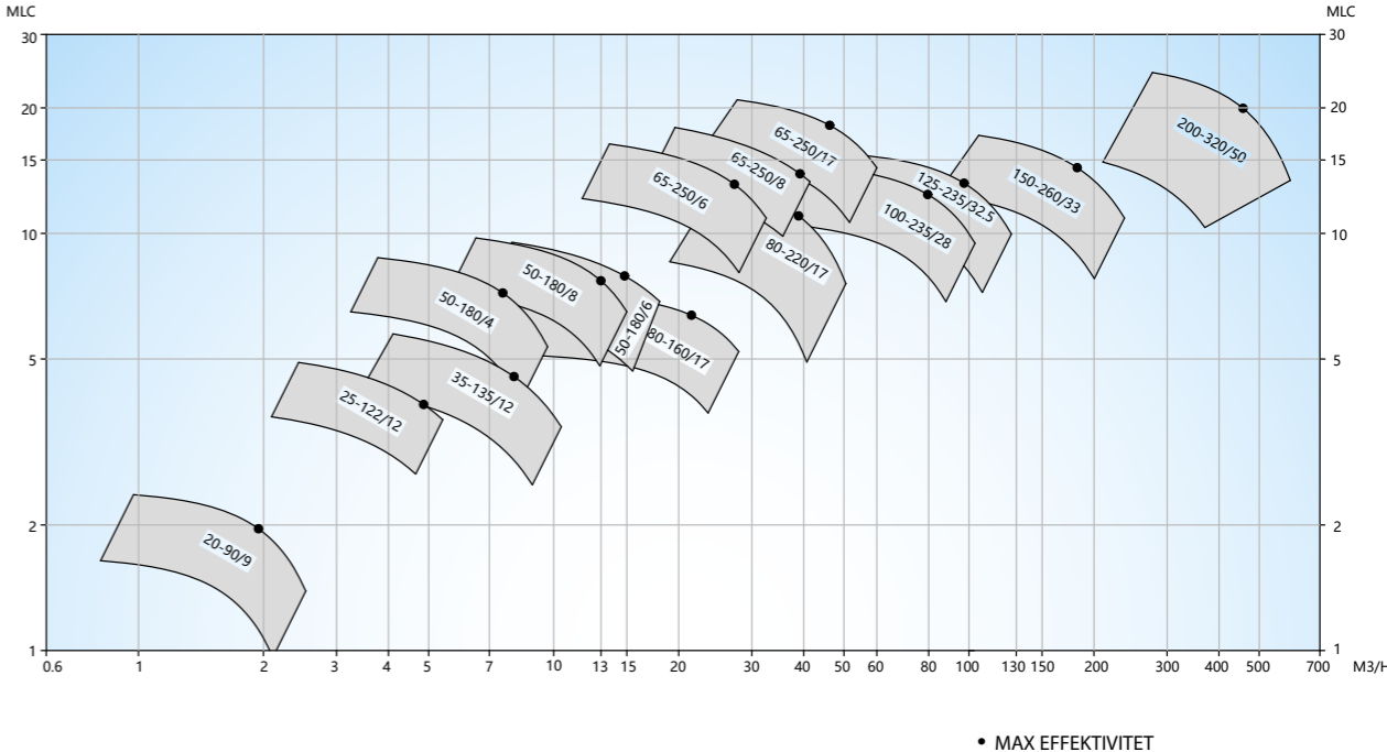
SA Centrifugalpumpe, 1450 o/min., 50 Hz
